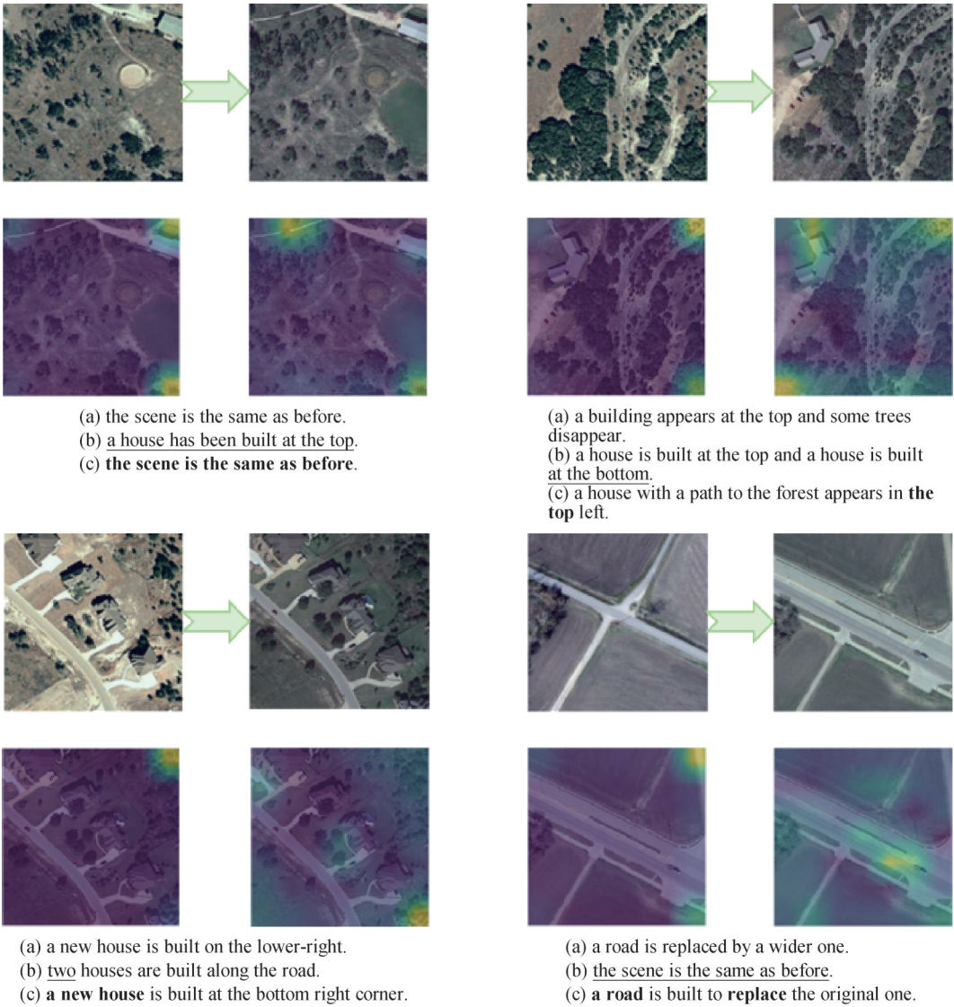
图2 典型样本的变化描述与注意力可视化对比结果
